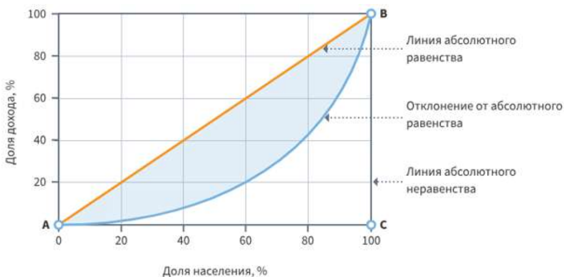
Рис. 2. Кривая Лоренца [8]
